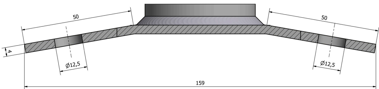
A-A ( 2:1 )
